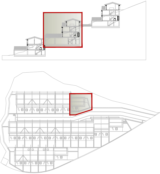
PLANTA PRIMERA
