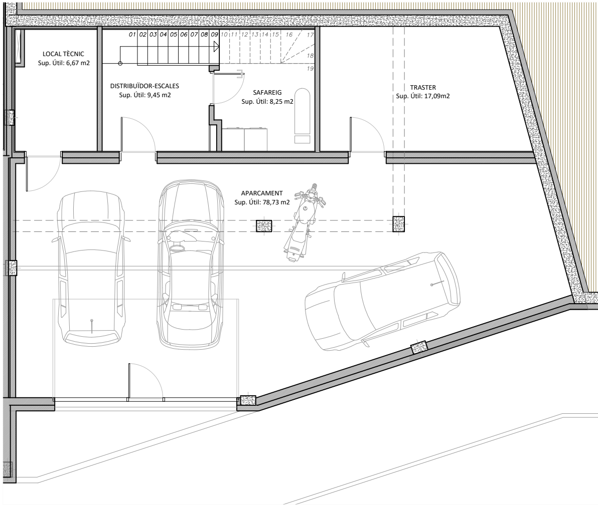
PLANTA SOTERRANI
