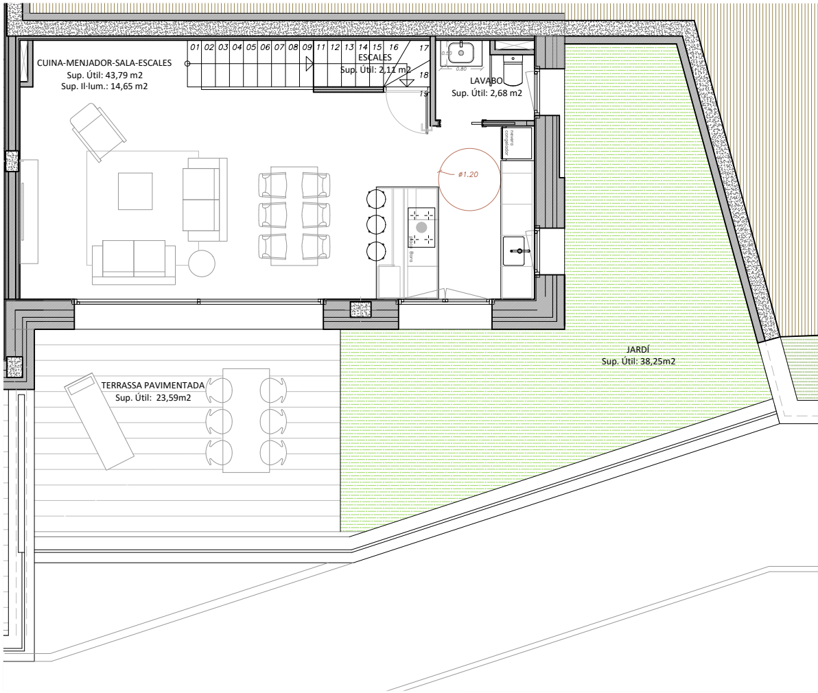
PLANTA BAIXA
